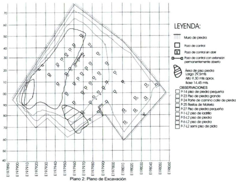
FIGURA 3: PLANO DE LA EXCAVACIÓN.
